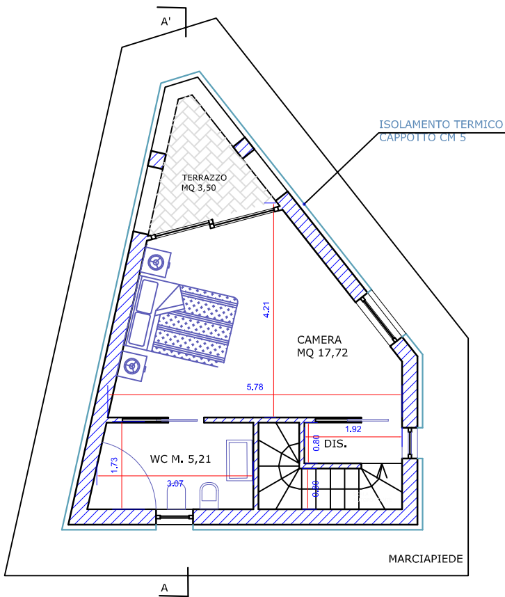
PIANTA P.P. H= 2,70 MT
