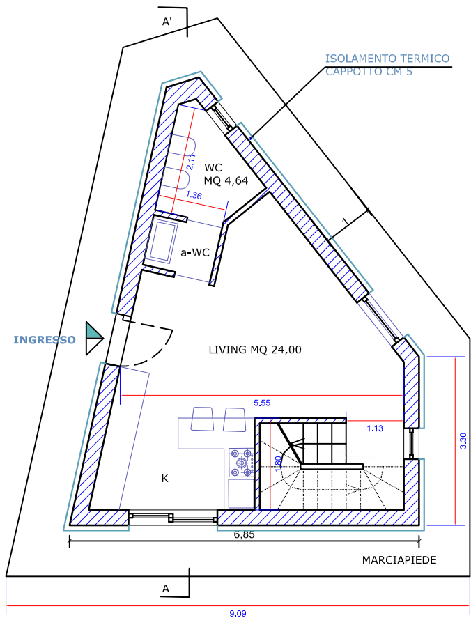
PIANTA P.T. H= 2,70 MT
