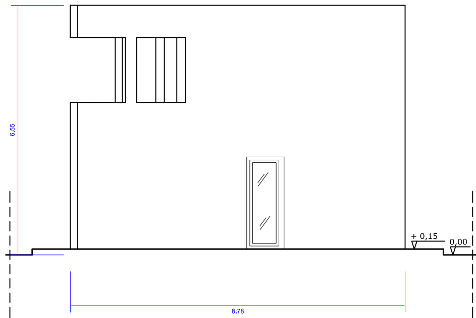
PROSPETTO OVEST
