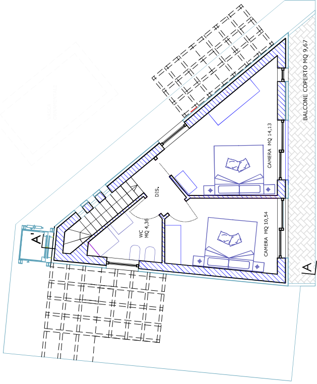
PIANTA P.P. H= 2,70 MT
