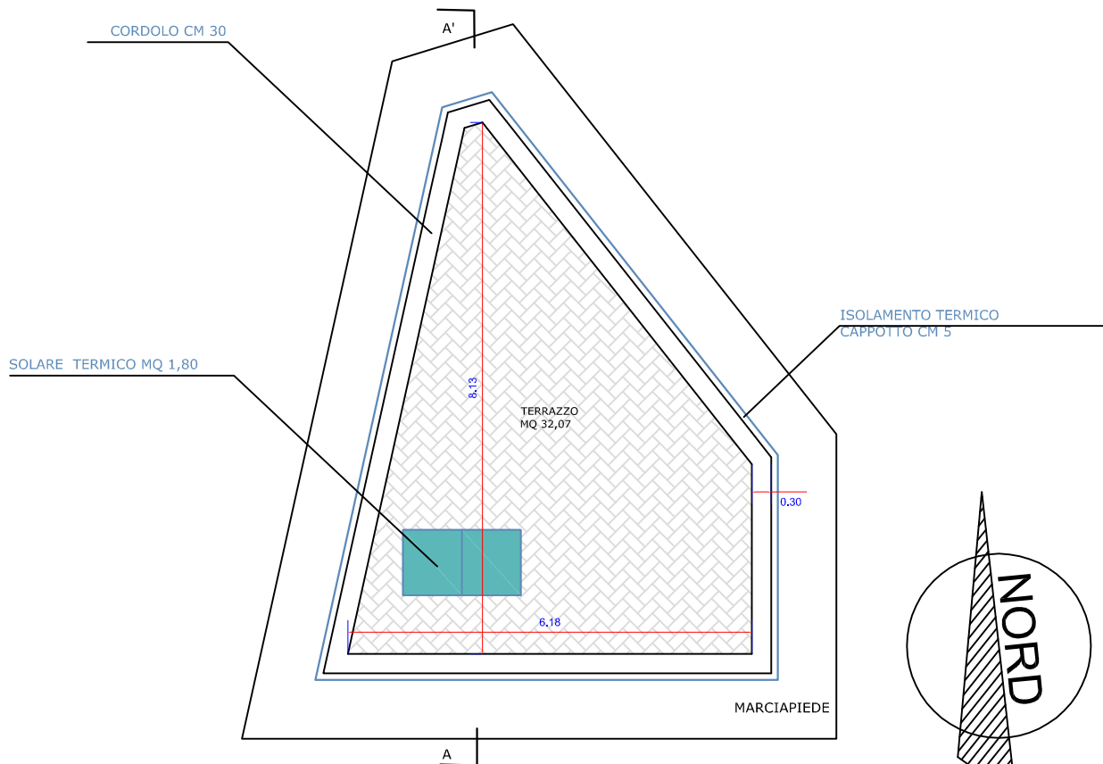
PIANTA COPERTURE TETTO PIANO NON ACCESSIBILE
