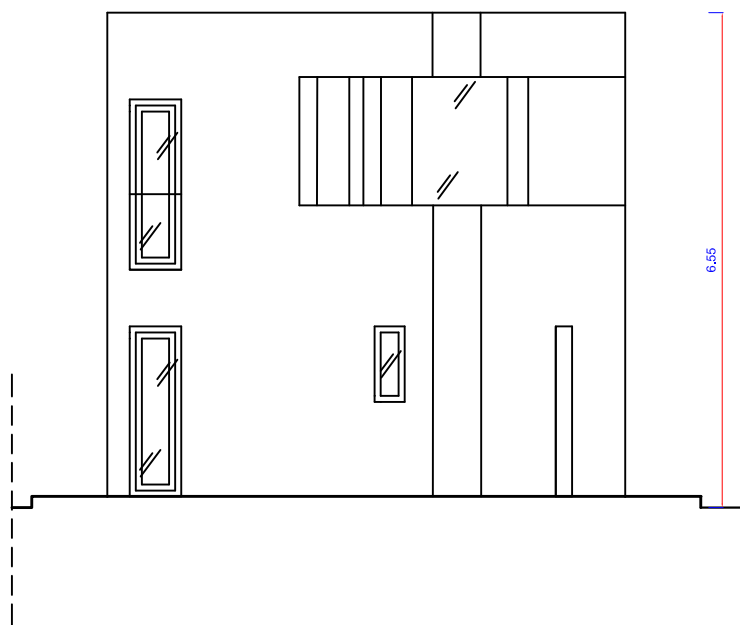
PROSPETTO NORD
